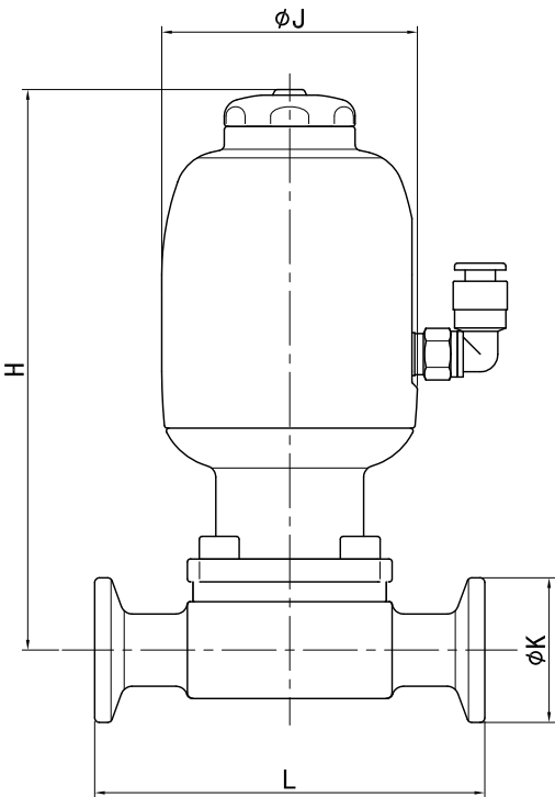
气动卡箍式
