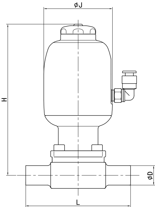
气动焊接式
